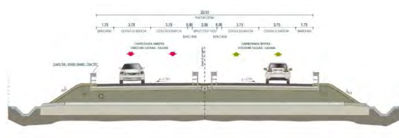
Figura B.2: Sezione tipo B del D.M. 5/11/2001 in rilevato
